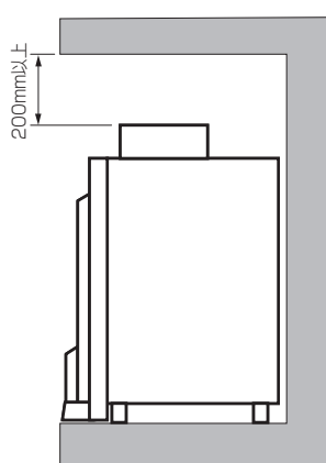
側面図 (Side View)
