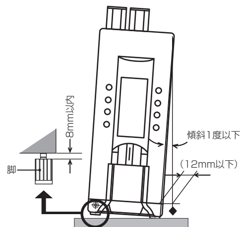
本機の傾き限界
